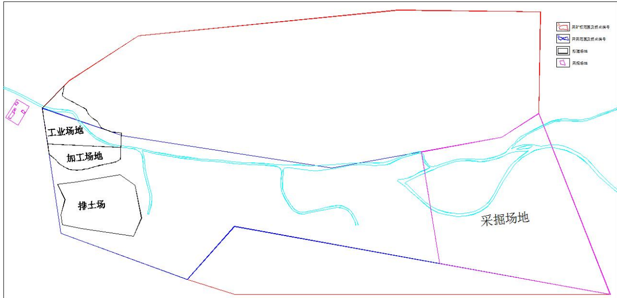
图 1-2 矿山平面布置示意图
