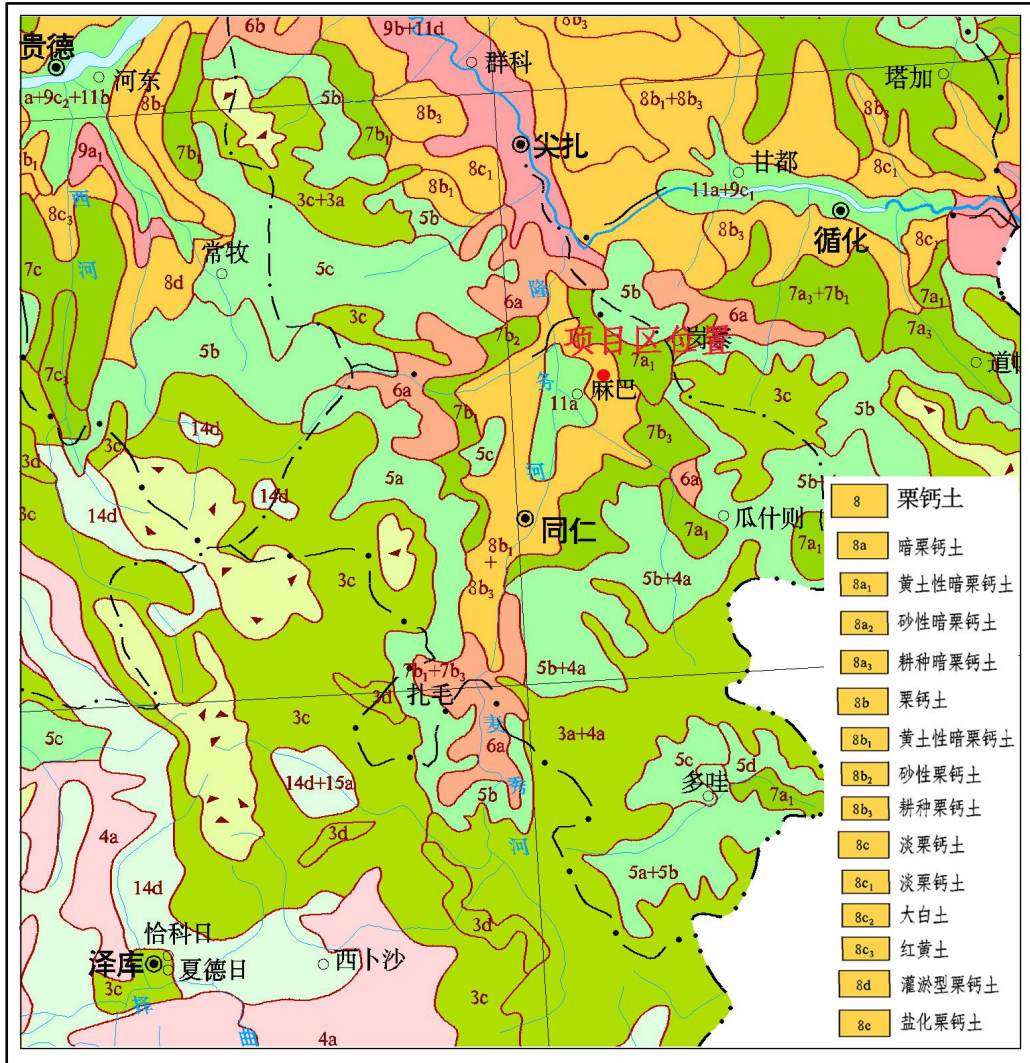
图 2-2 矿区土壤类型图
