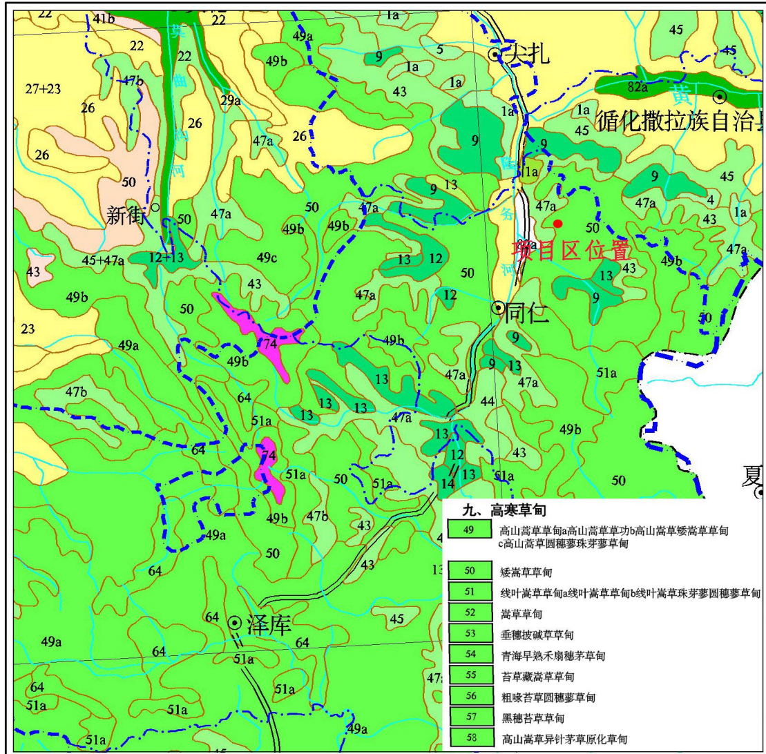
图 2-1 矿区植被类型图
