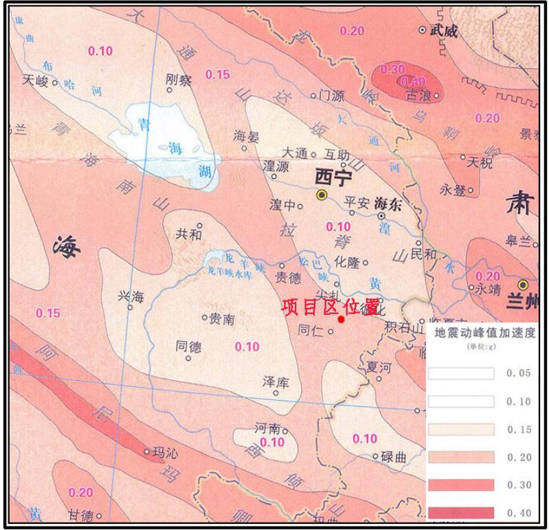
图 2-3 中国地震动峰值加速度区划图
