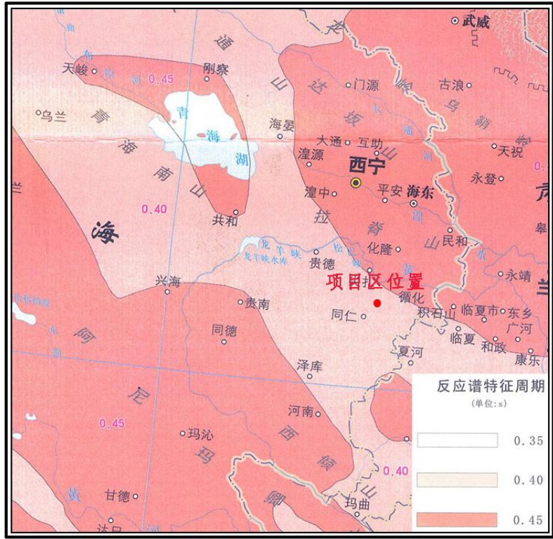
图 2-4 中国地震动加速度反应谱特征周期区划图
